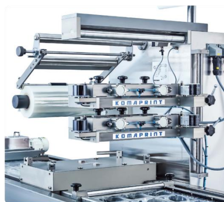
<スマート・マルチラベラー>
