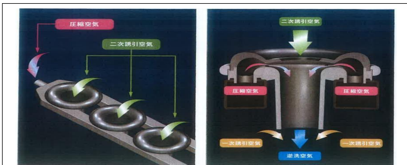
<CK インジェクターの原理：コアンダ効果の応用>
